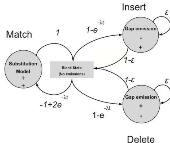
Fig. 1. Bogusz & Whelan. 2017. Syst. Biol. 66(2):218–231
