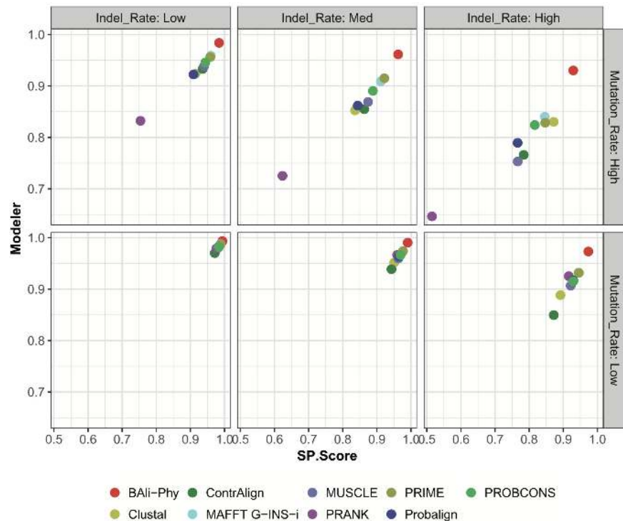
Fig. 6. Nute et al. 2018. Syst. Biol. https://doi.org/10.1093/sysbio/syy068
